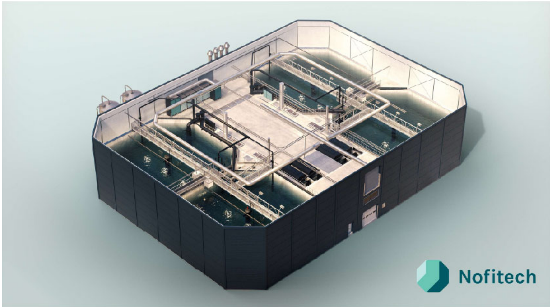
Figur 1: Resirkuleringsanlegg fra Nofitech. Et 45 x 33 meter stort anlegg inneholder fire tanker på 16 meter i diameter og er typisk dimensjonert for å fôre opp til 3 tonn fôr per dag. Illustrasjon: Nofitech.
